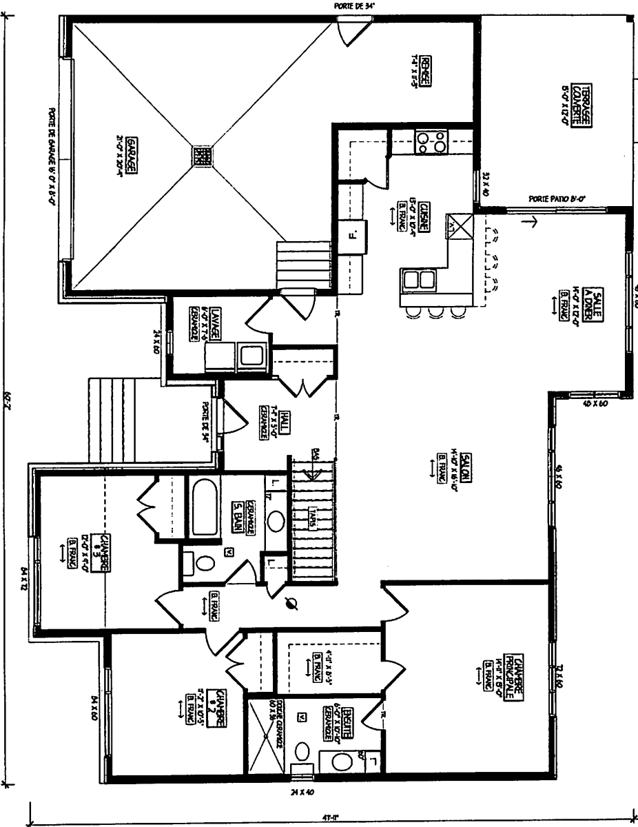
PLAN DE REZ DE CHAUSSEE
