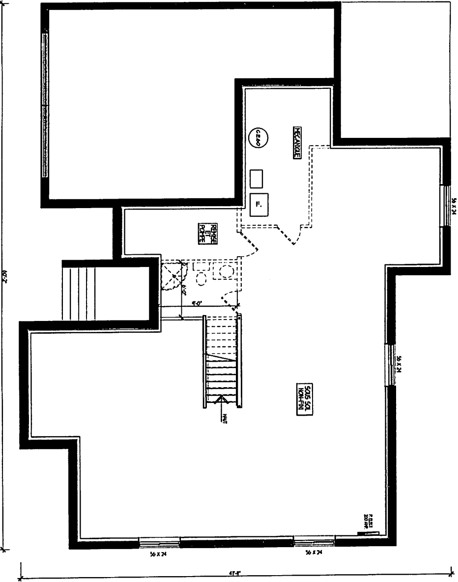
PLAN DE SOUS SOL NON FINI
